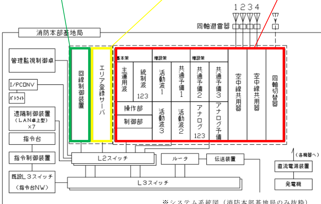
※システム系統図 (消防本部基地局のみ抜粋)
